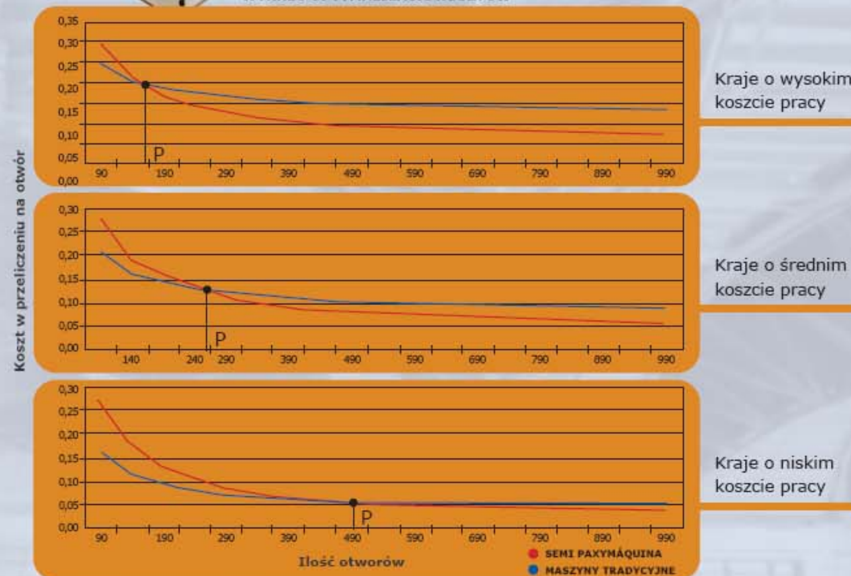
P: Miejsce przecięcia się kosztów maszyny tradycyjnej i SEMI PAXY.
